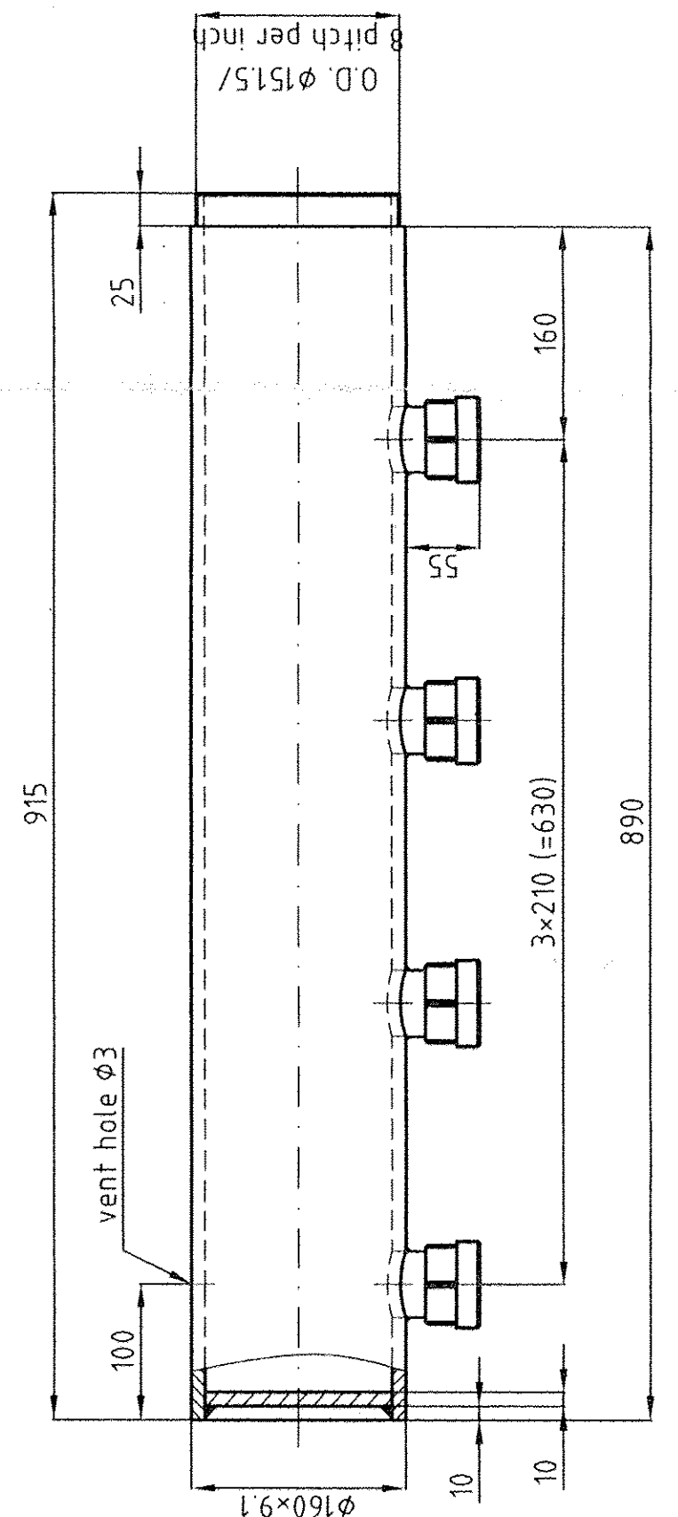
pos. 4.1 1:5
