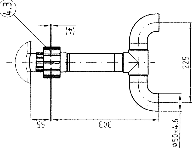
Pos. 4.2 1:5
