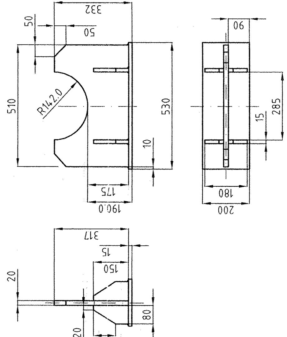
pos. 5.2
