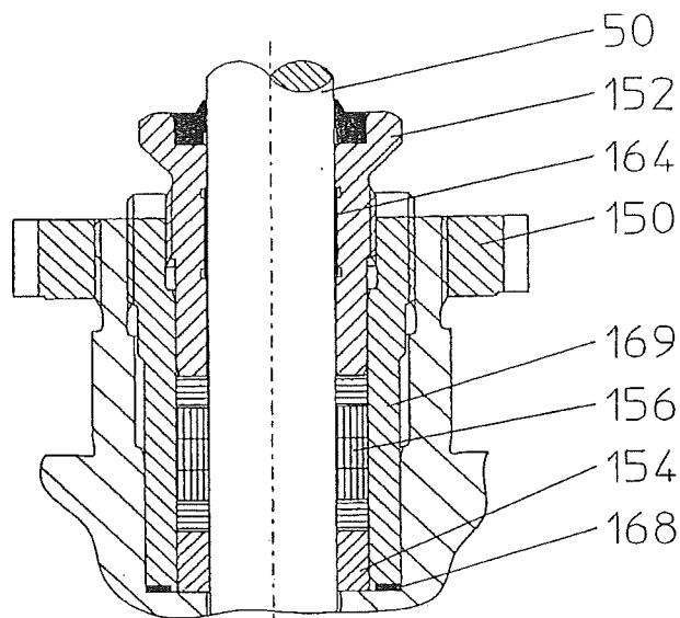
Detail X - Spindelabdichtung
