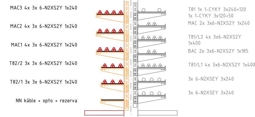
Detail uloženia káblov na existujúcom káblovom moste M1:50
